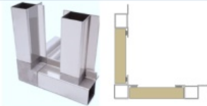
Каркасный корпус 25 мм
