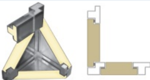
Каркасный корпус 50 мм
