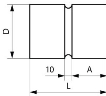
Ниппель наружный
