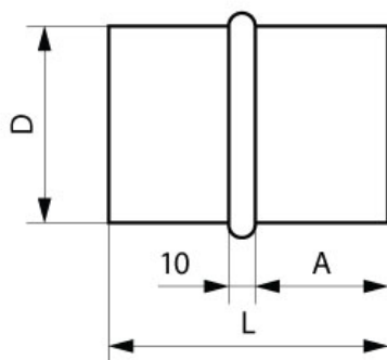
Ниппель внутренний
